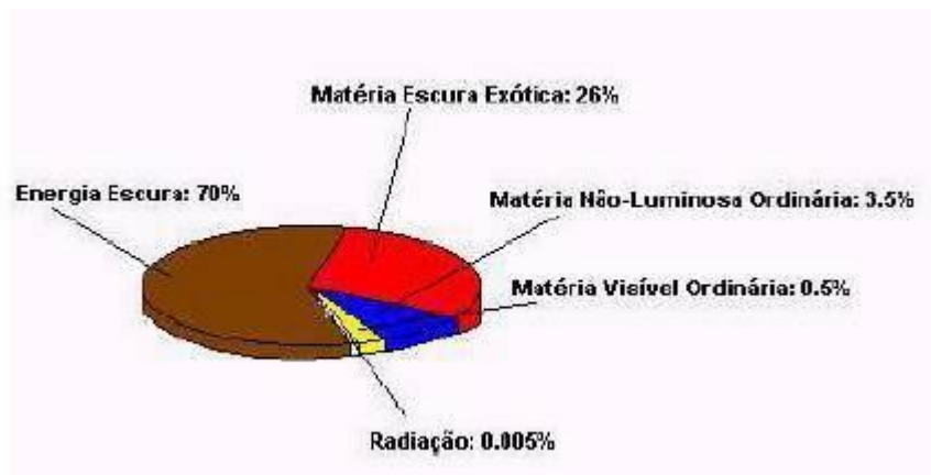
Figura 1: Os ingredientes do Universo em sua constituição aproximada.
